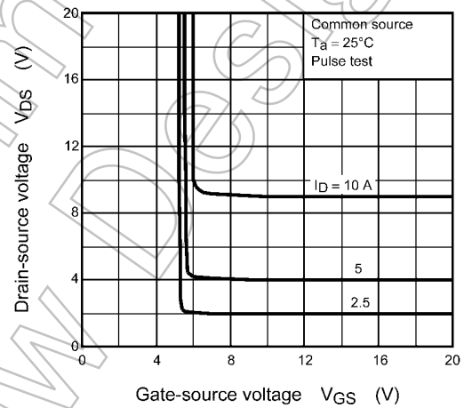
Fig. 8.4 V_{DS} - V_{GS}
